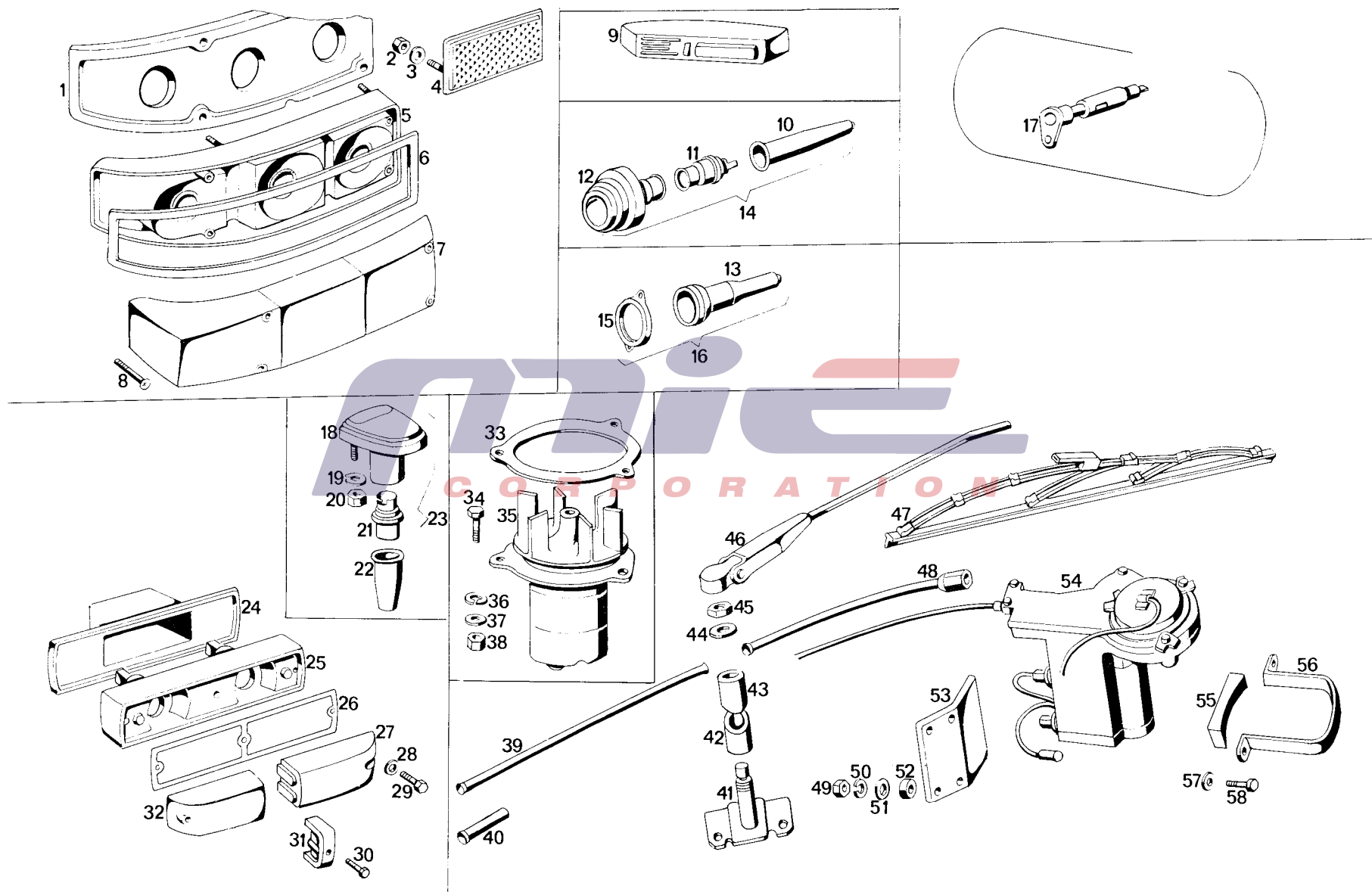
TAVOLA 3-EQUIPAGGIAMENTO ELETTRICO TABLE 3-ELECTRIC EQUIPMENT
