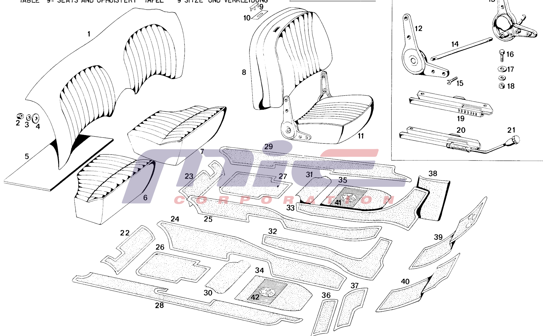
TAVOLA 9- SEDILI E RIVESTIMENTI TABLEAU 9 SIEGES ET RECOUVREMENT TABLE 9- SEATS AND UPHOISTERY TAFEL 9 SITZE UND VERKLEIDUNG
