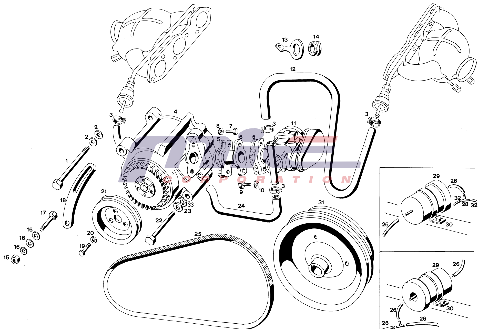
Tavola 5 - Pompa aria Table 5 - Air pump
