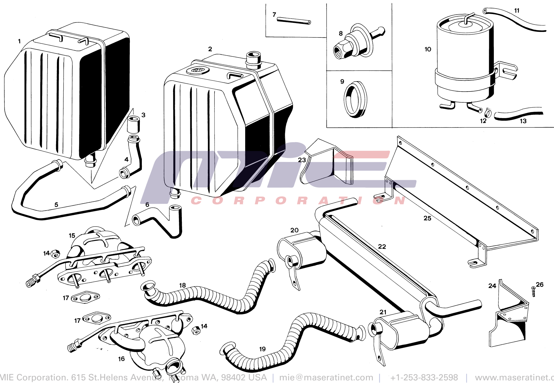
Tavola 8 - Serbatoi benzina - Tubo di scarico Table 8 - Fuel tank - Exhaust pipes
