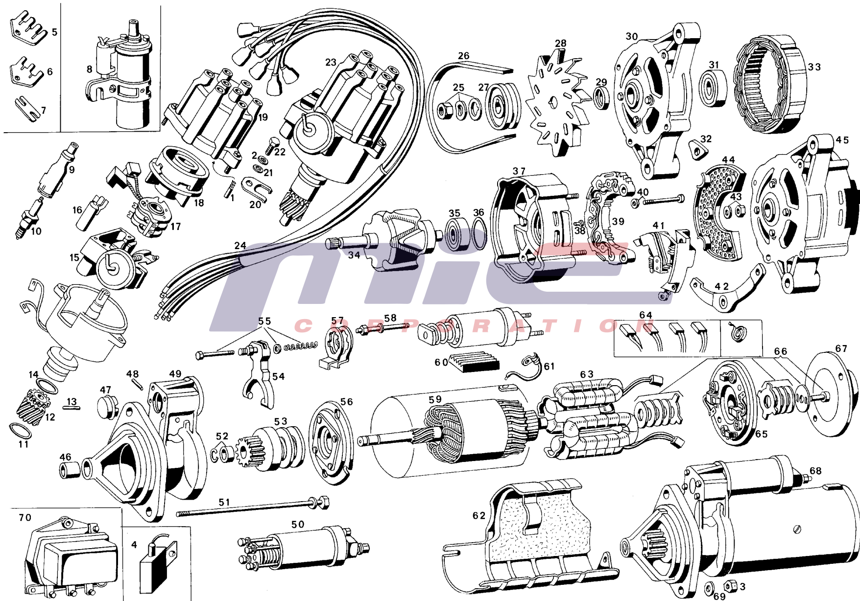
Tavola 7 - Equipaggiamento elettrico Table 7 - Electrical equipment
