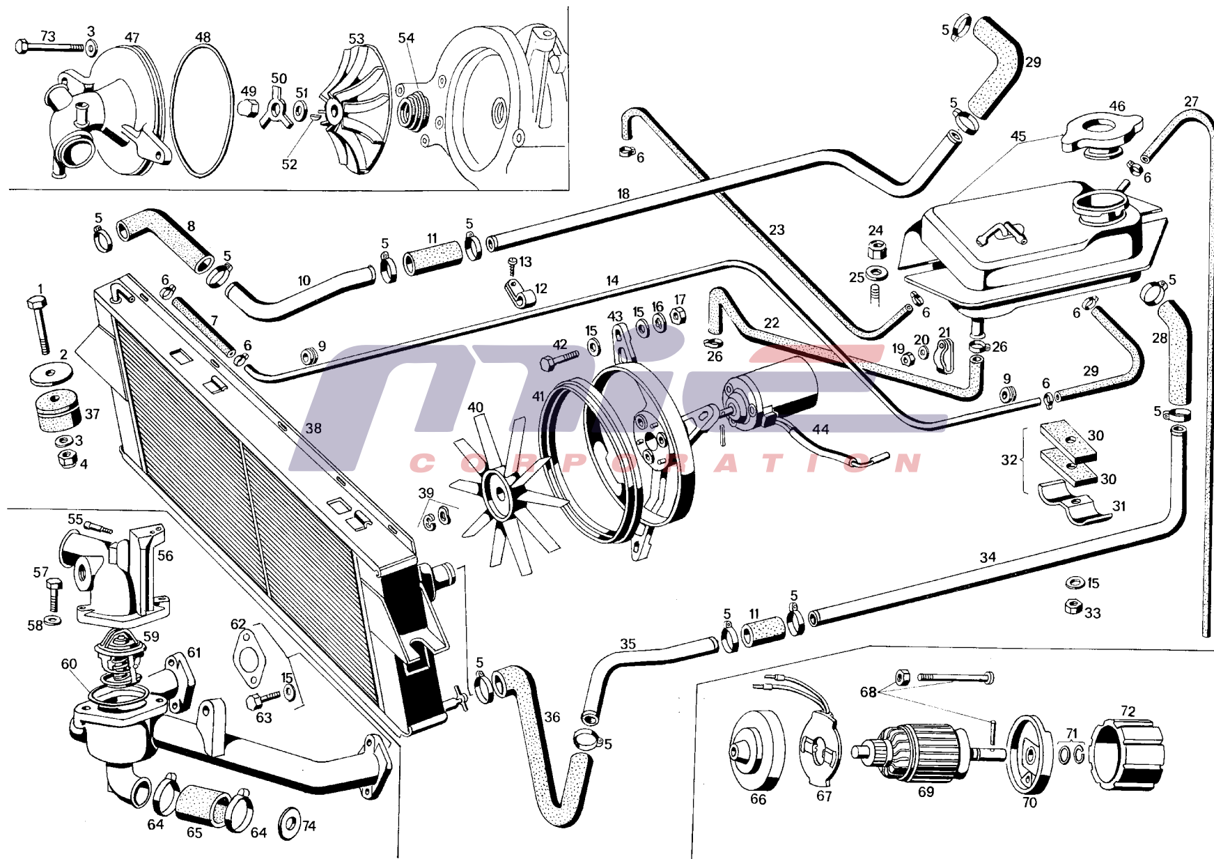
Tavola 6 - Raffreddamento del motore Table 6 - Engine cooling
