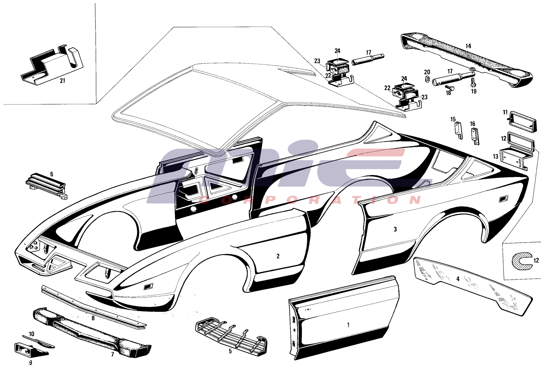
Tavola 9 - Scocca anteriore Table 9 - Front body
