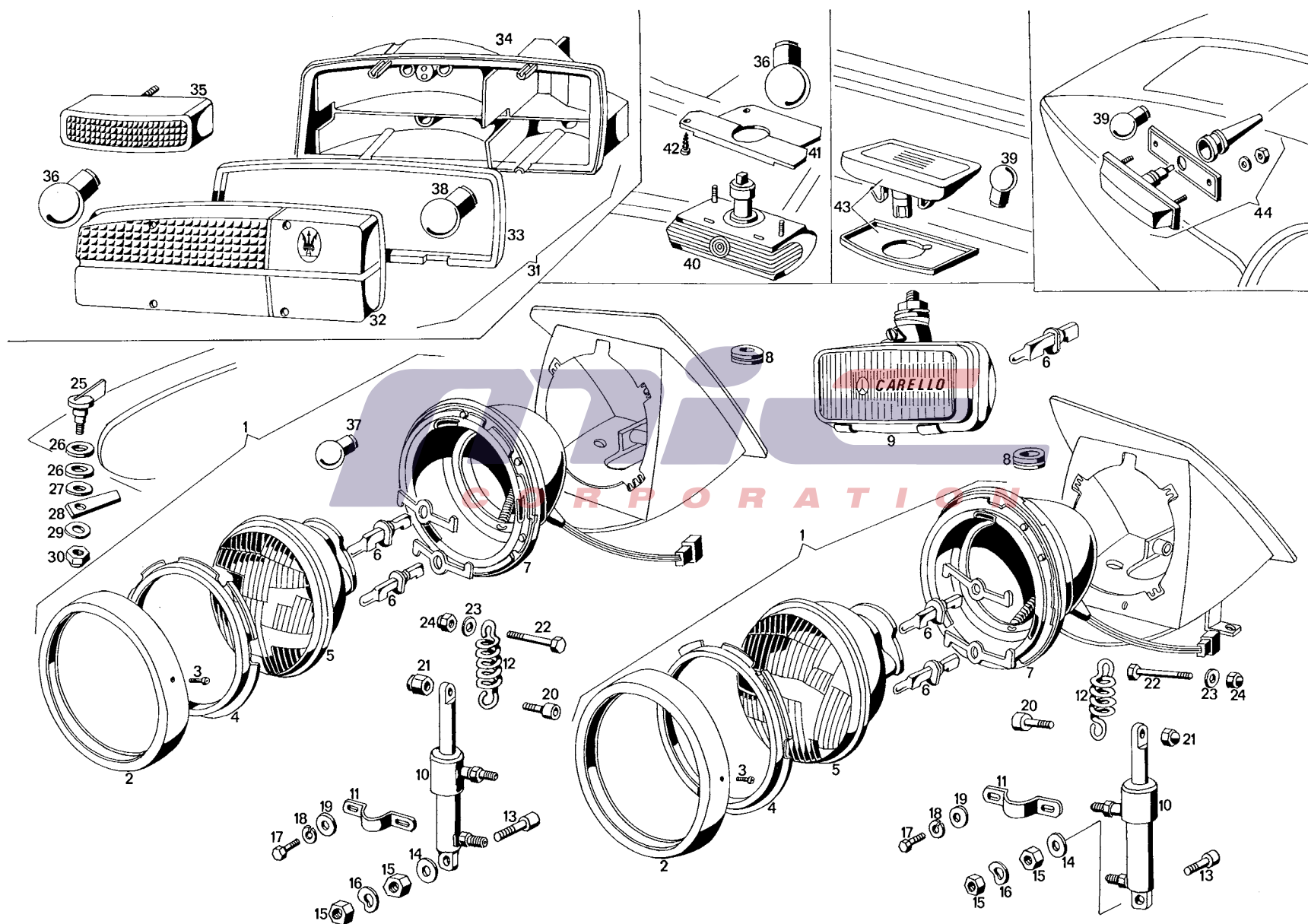
Tavola 29 - Fanaleria Table 29 - Lights
